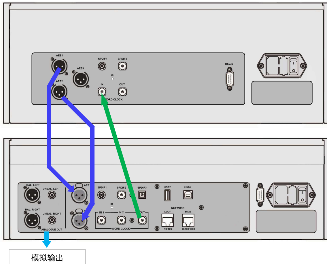
图 2 – 在主模式下将 Rossini Player 与 Transport (CD / SACD 转盘激光唱机) 一起使用
