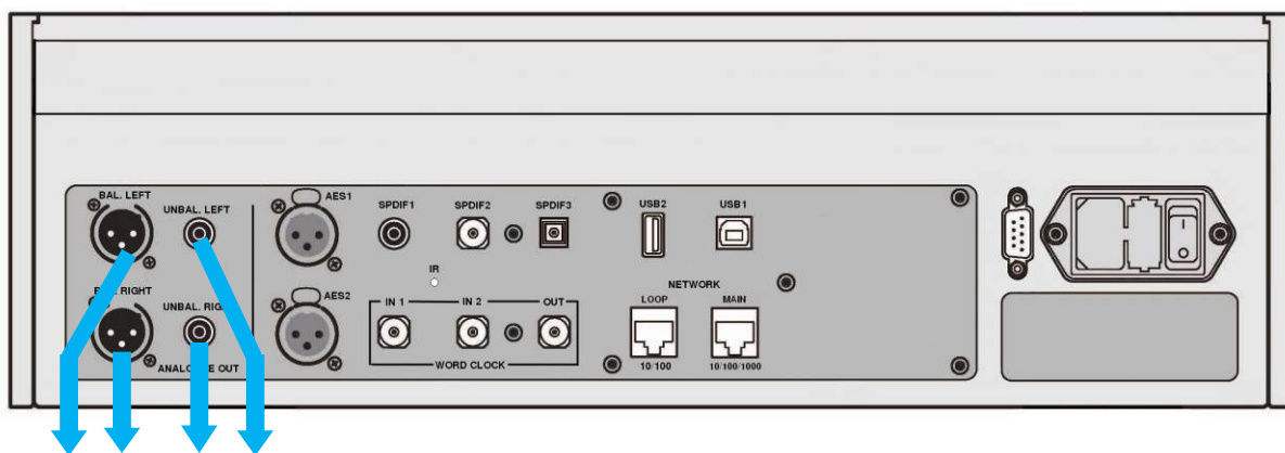
图 1 – Rossini Player 的基本设置
