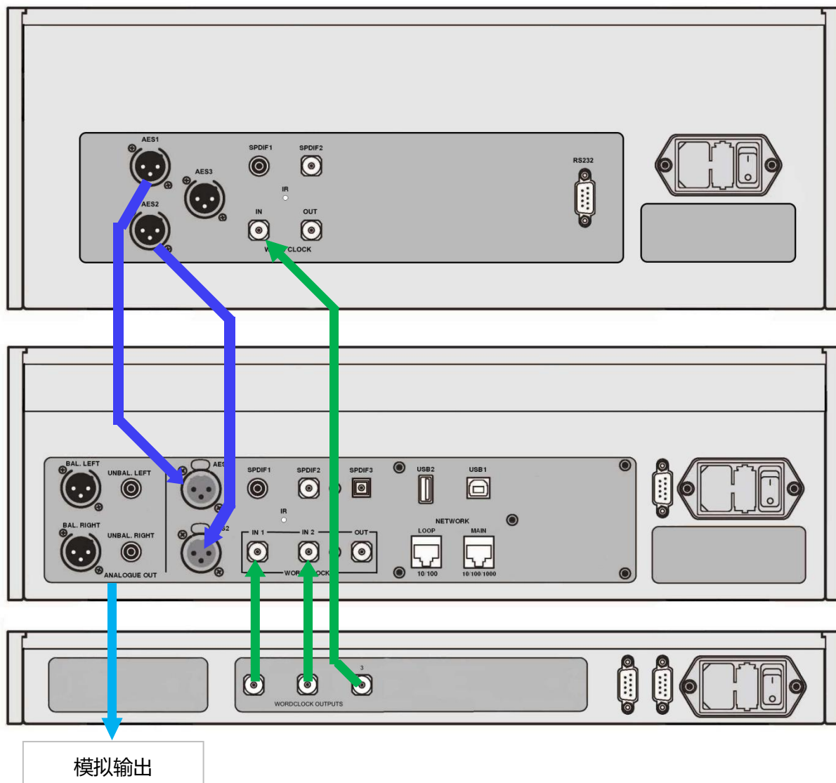
图 3 – 将 Rossini Player 和 Clock（音频时脉校准机）与 Transport（Rossini CD / SACD 转盘激光唱机）一起使用
